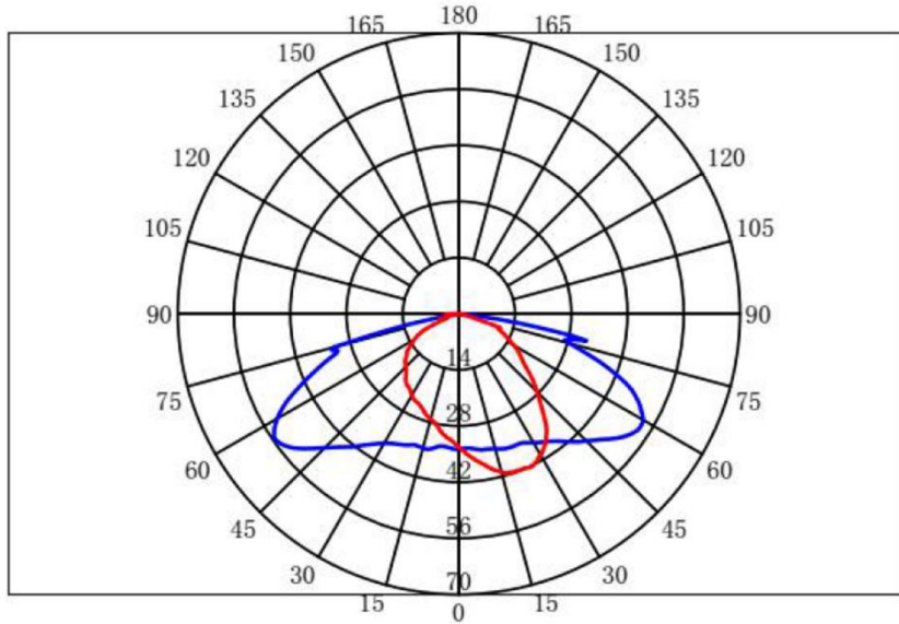
配光曲线
