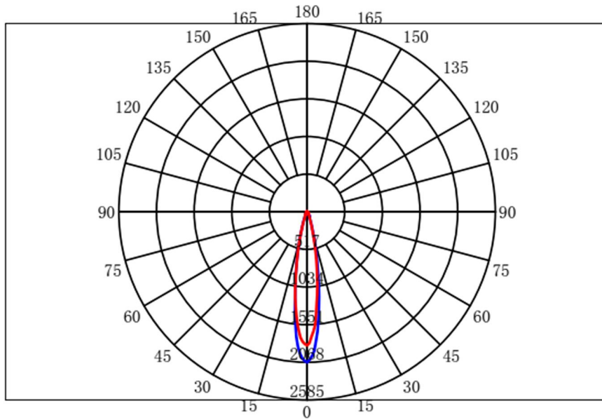
配光曲线
