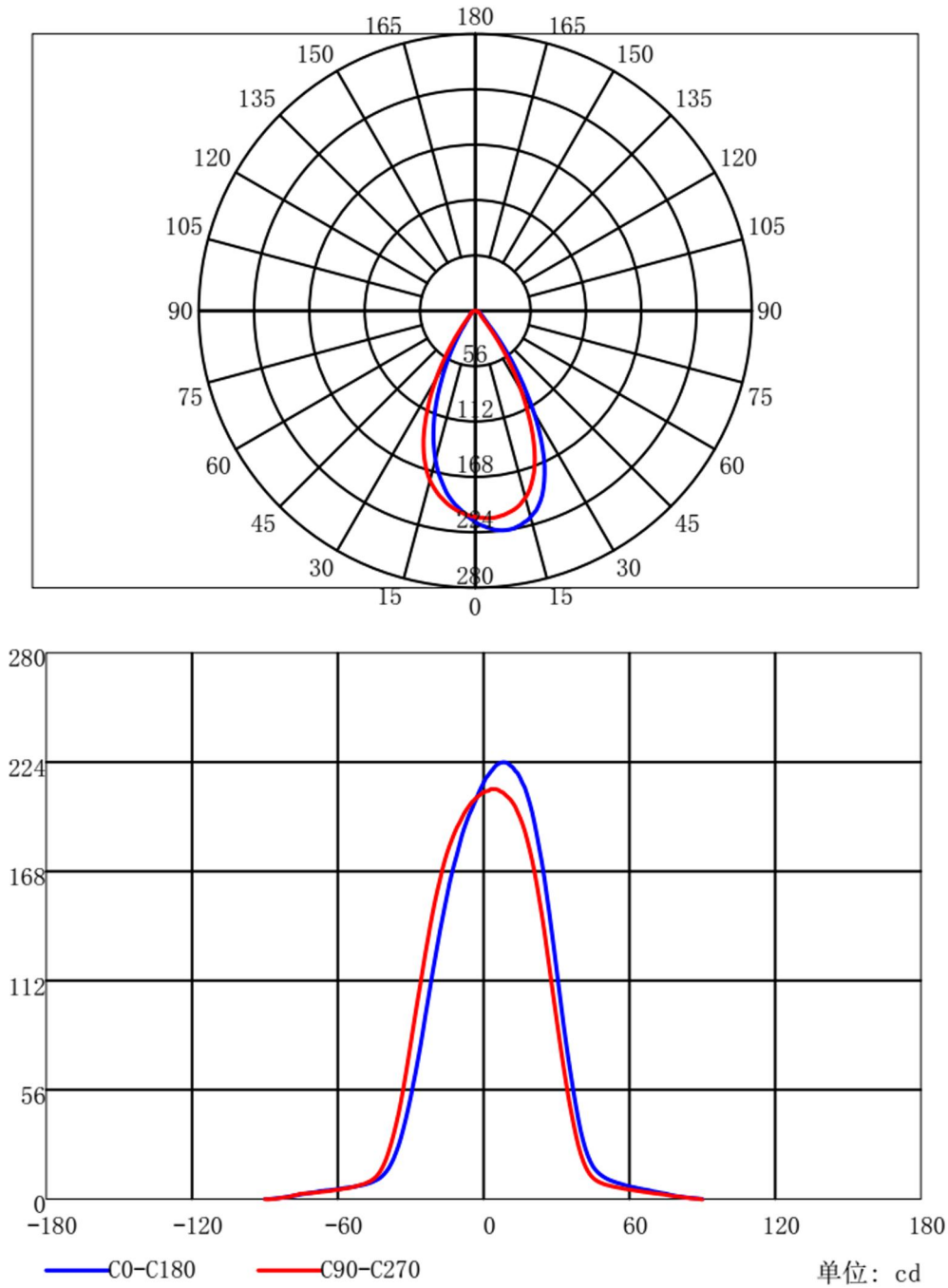
配光曲线
