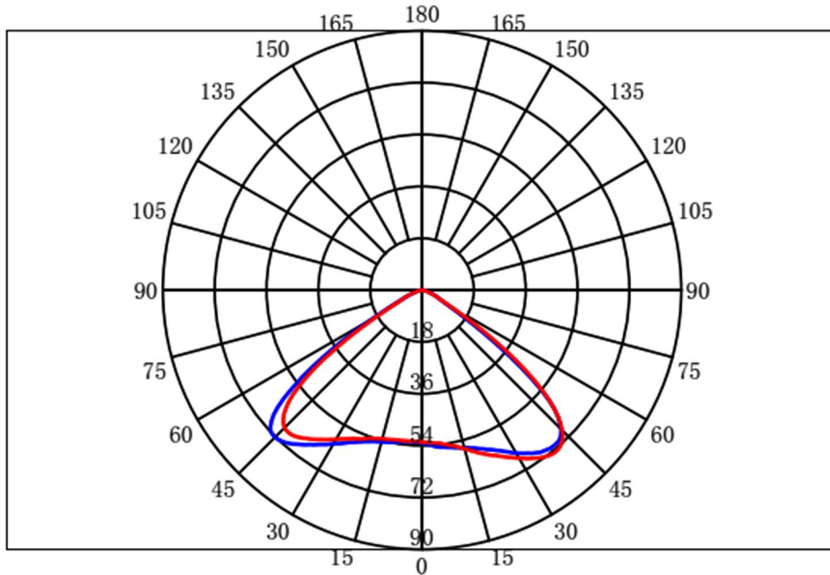
配光曲线
