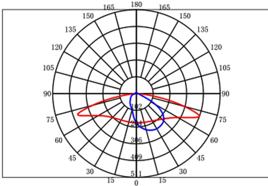
配光曲线
